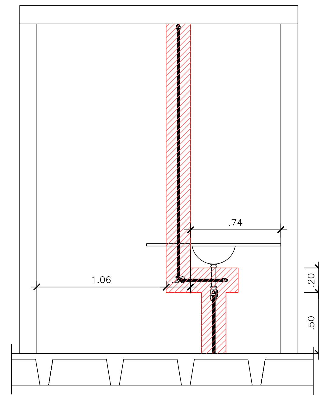
Vista J ESCALA 1/25
