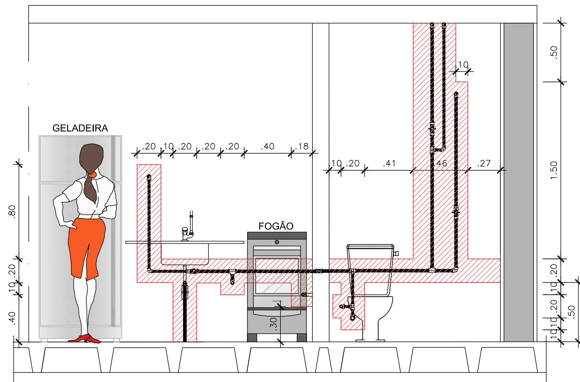
Vista I ESCALA 1/25
